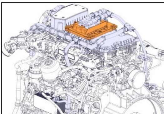
Bộ điều khiển EMS (A14)
